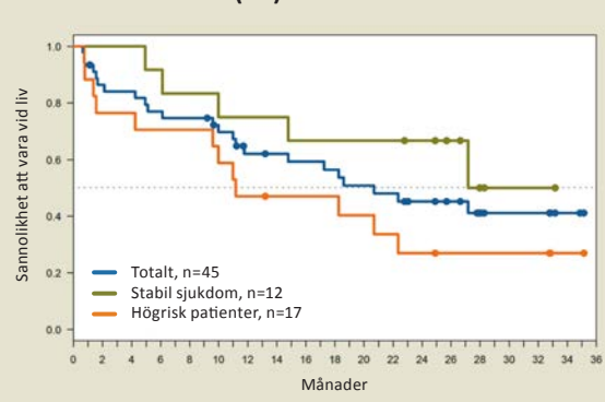
Medianöverlevnad (OS)
